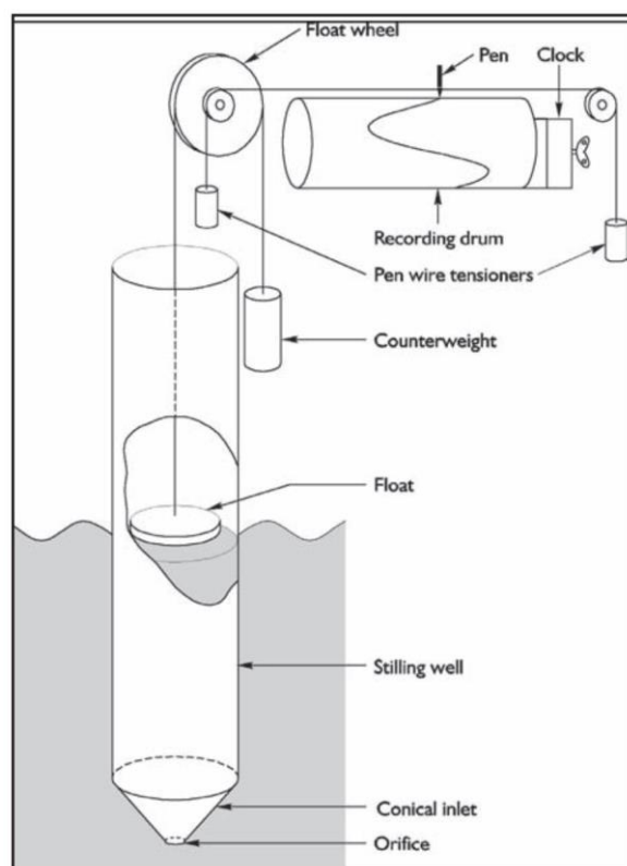
سیستم دستگاه جزر و مد سنجی شناوری
