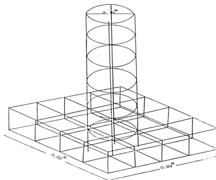
آرماتوربندی ایستگاه ژئودزی درجه صفر از نوع پیلار
