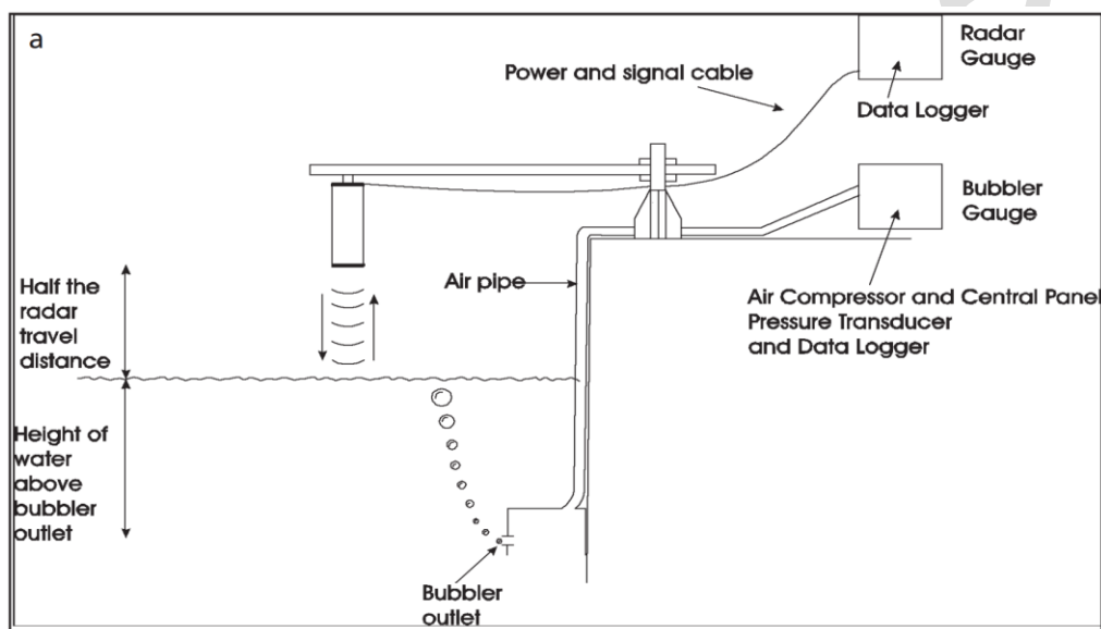
تایدگیج راداری به همراه سنسور فشاری حبابی
