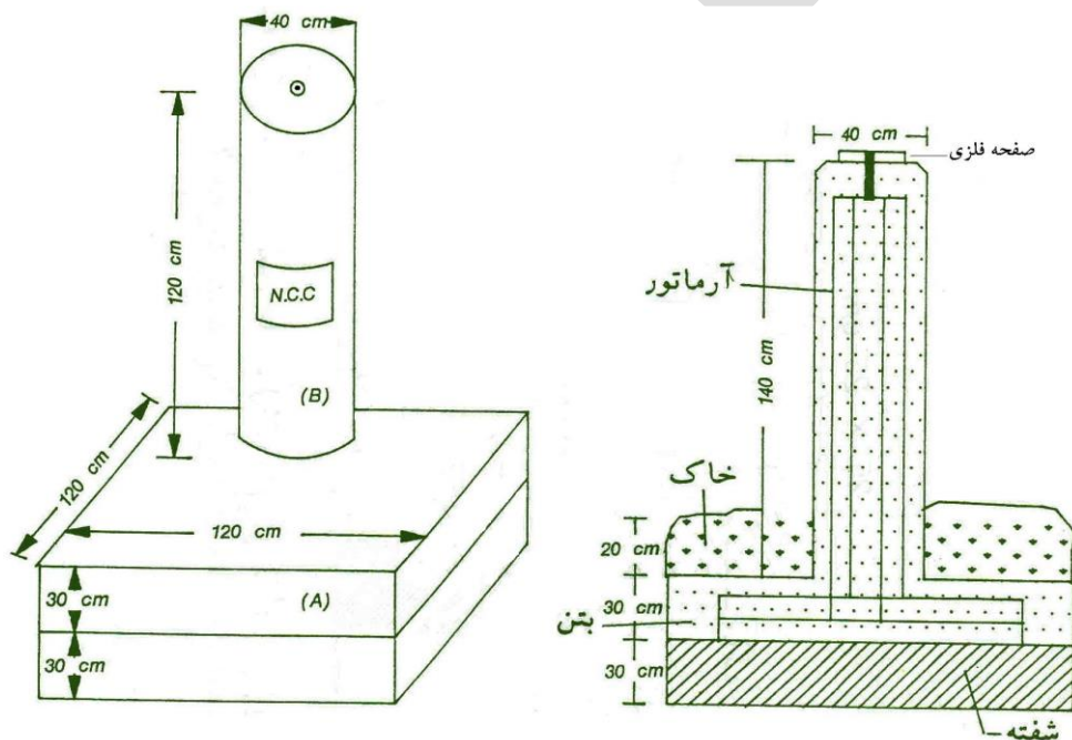
ساختمان ایستگاه ژئودزی درجه صفر از نوع پیلار
