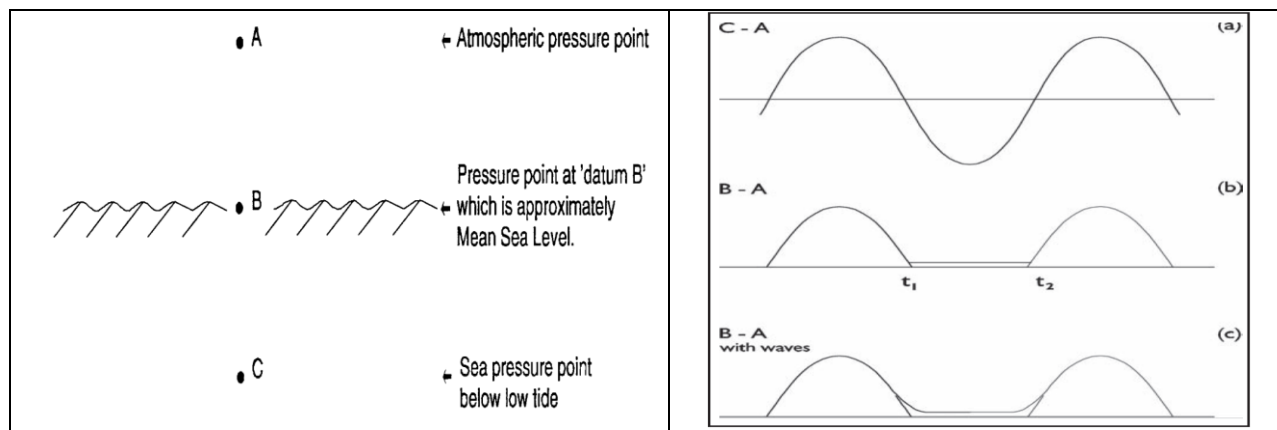
محل نسبی سنسورهای فشاری در نوع B و نمودارهای مشاهدات و اختلاف مشاهدات
