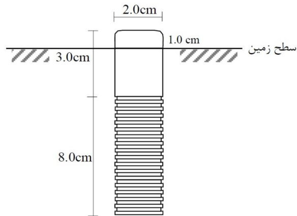
میله ترازبایی سرگرد مورد استفاده در ساختمان سنگی و بتنی
