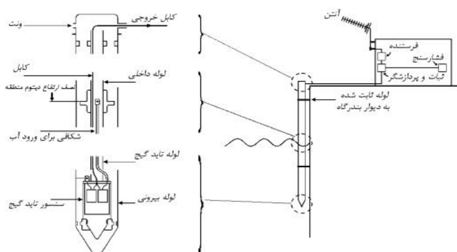
سنسور فشاری مشاهده مستقیم
