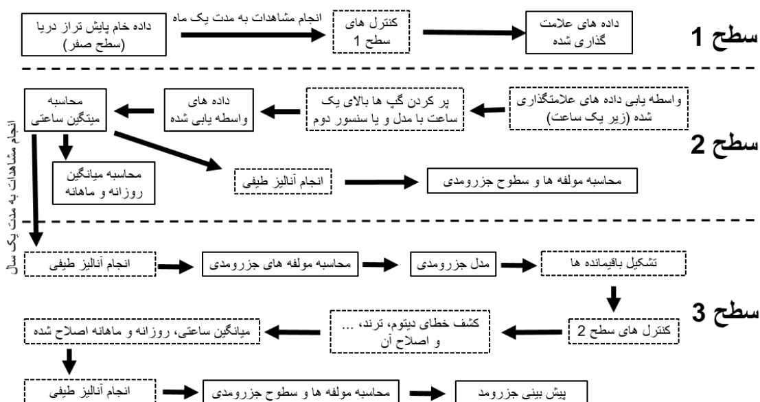
شکل 7-1 فرآیند کلی پردازش داده های تراز دریا
